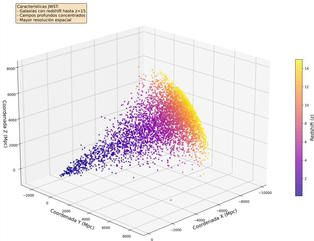
Distribución 3D de 5000 Galaxias - Datos JWST (Simulación)
