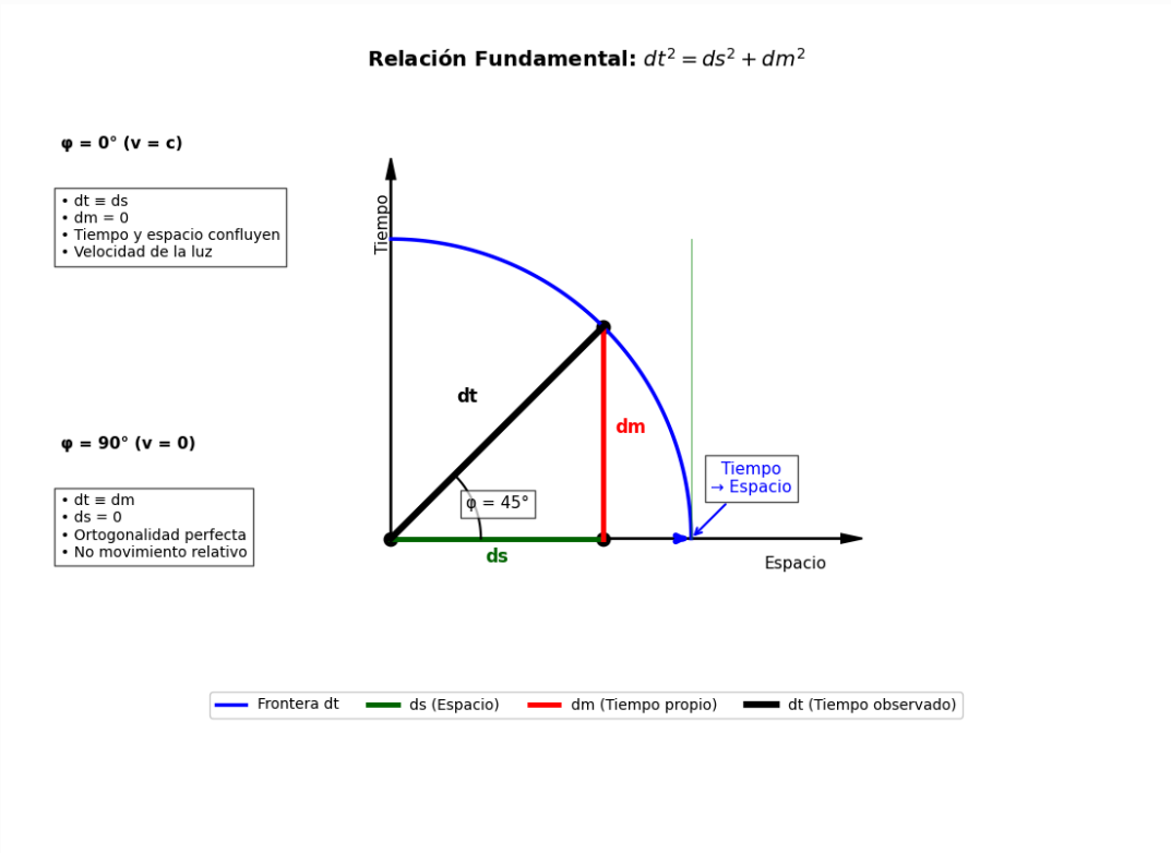
Figure 1 : espace-temps
