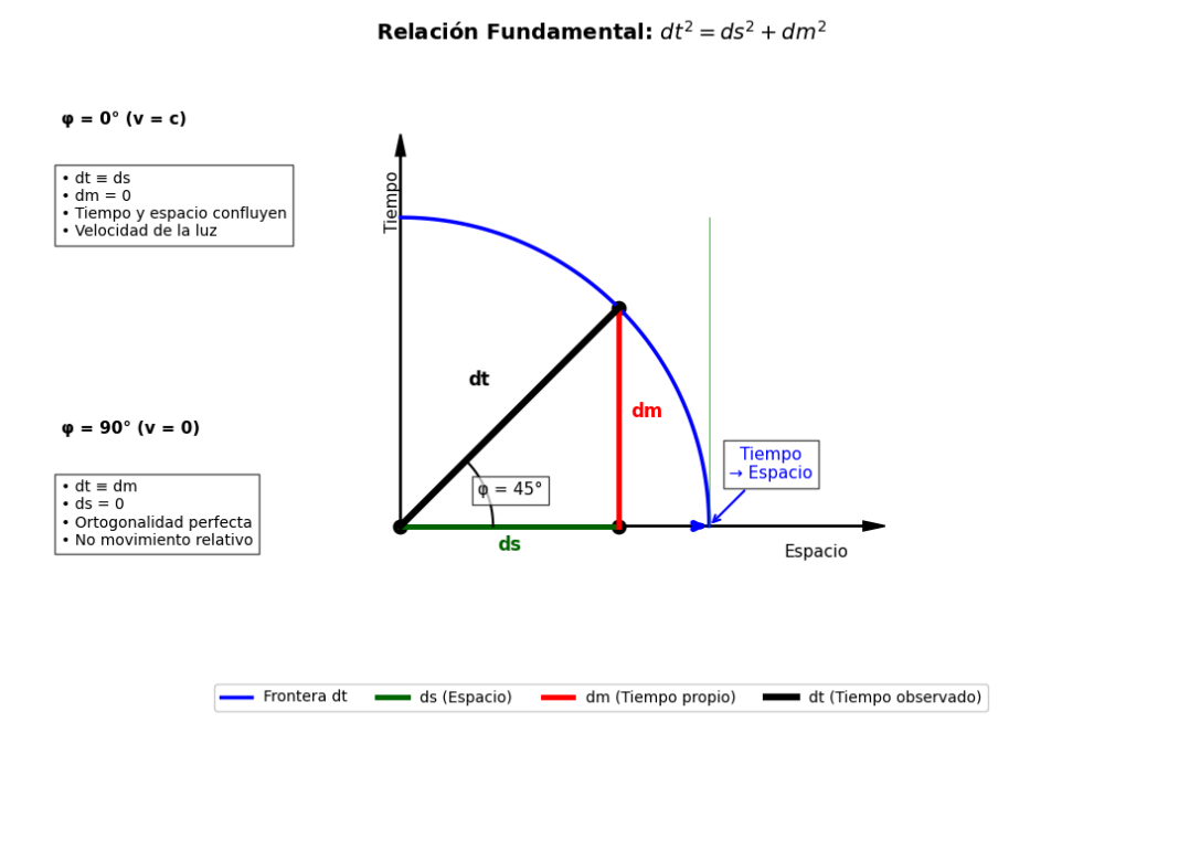
Figure 1: espacio-tiempo
